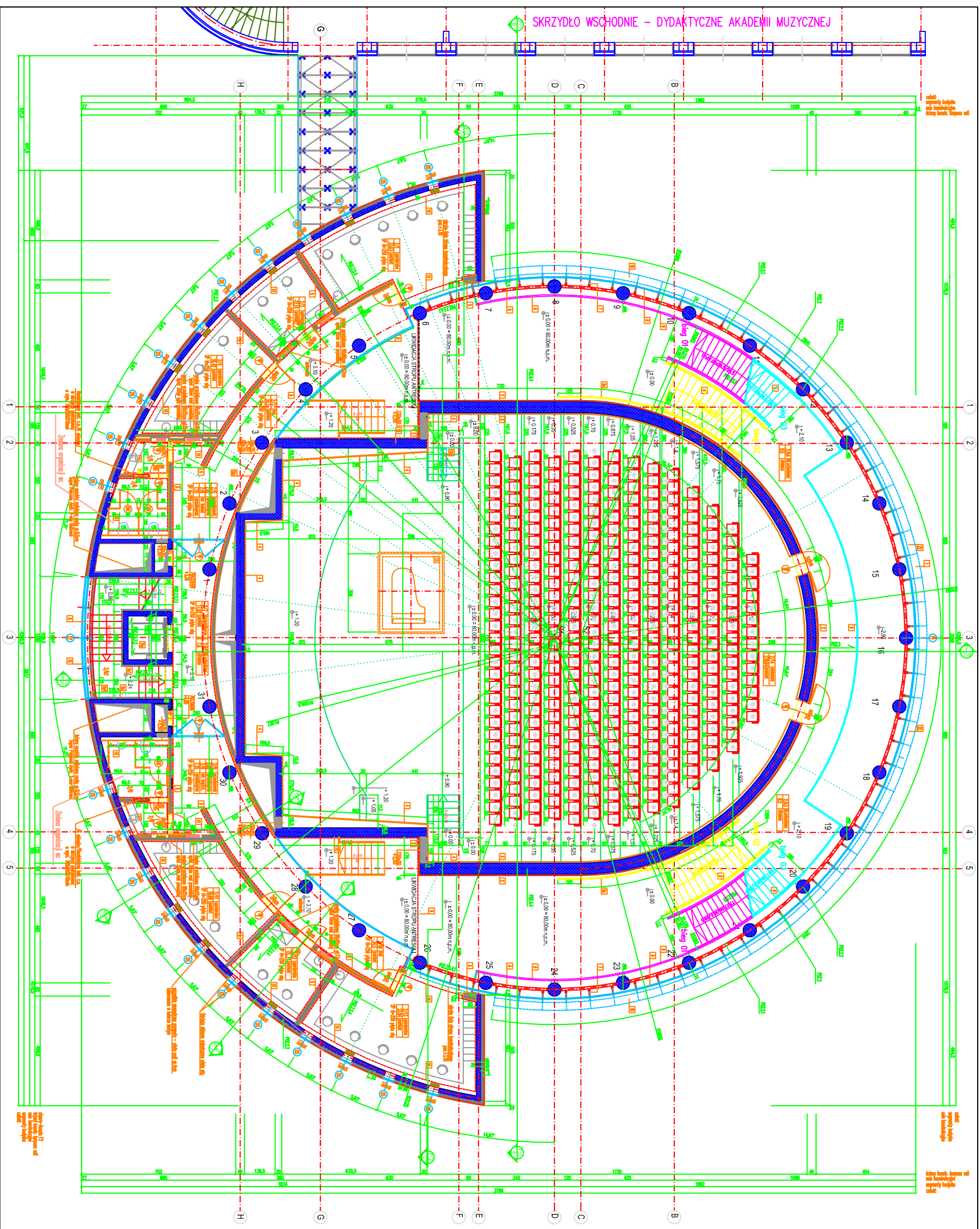
SALA KONCERTOWA AKADEMII MUZYCZNEJ IM IGNACEGO JANA PADEREWSKIEGO W POZNANIU RZUT POZIOMU +2.10 / +3.10
