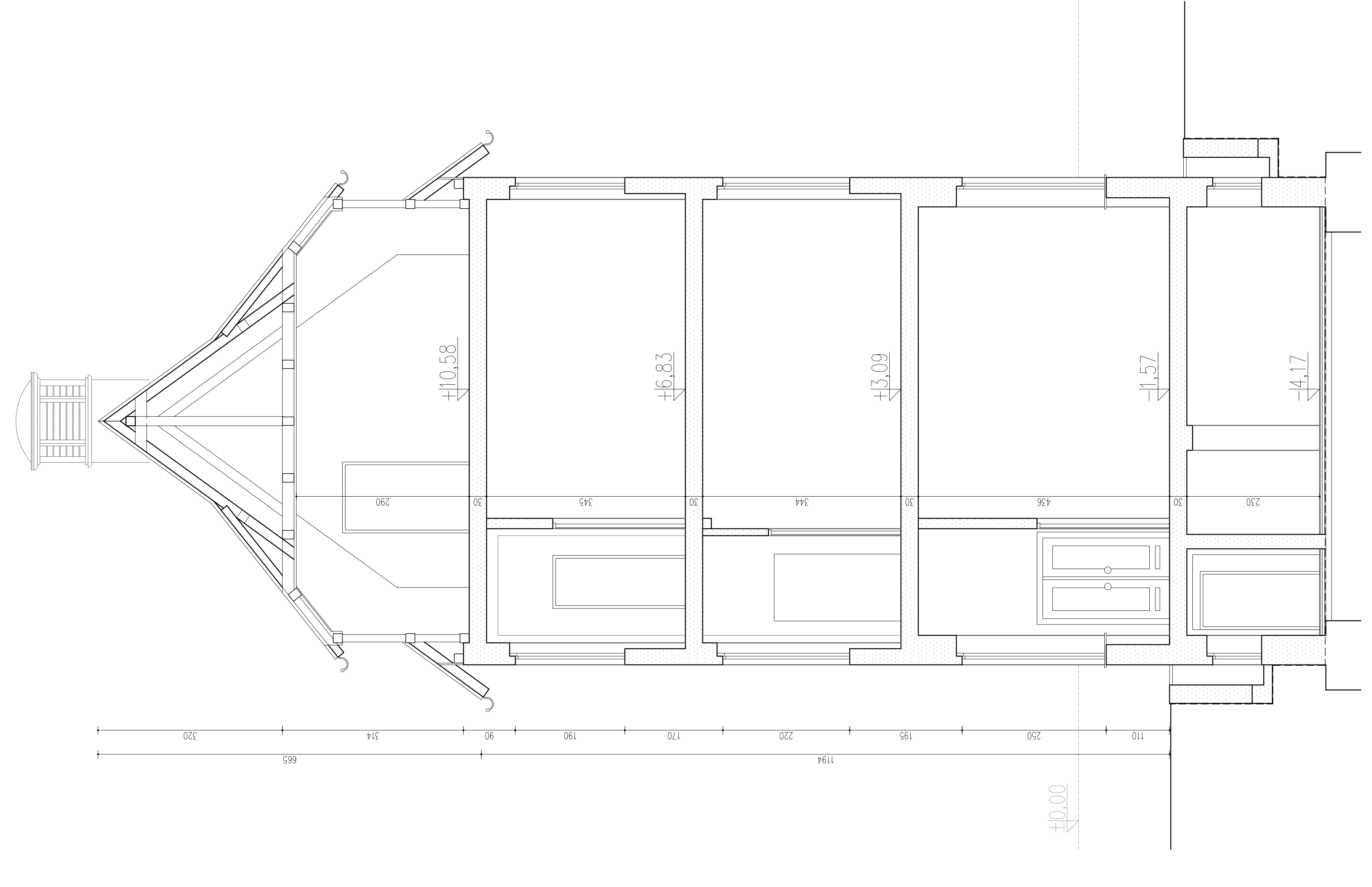
PRZEKRÓJ C-C
